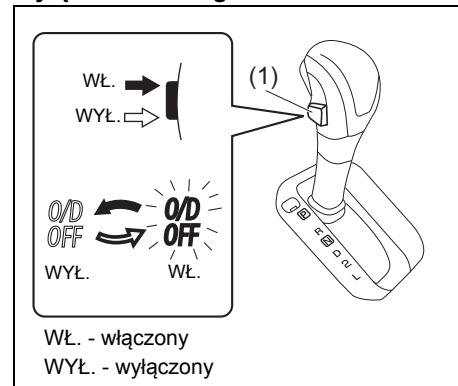
(1) Wyłącznik nadbiegu
